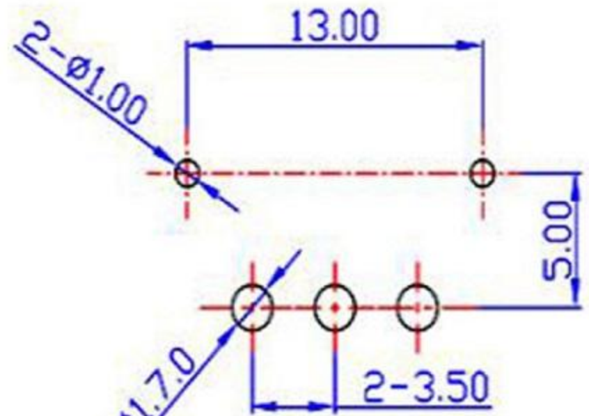
安装孔示意图
